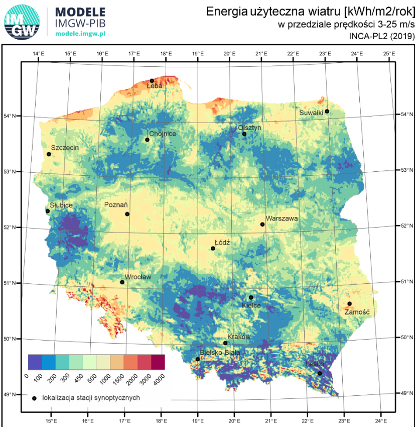
Rysunek 11. Średnia roczna suma energii wiatrowej [kWh/m²/rok] na poziomie 10 m n.p.g. na terenie otwartym na obszarze Polski w 2019 roku Źródło: Atlas Małej Energetyki Wiatrowej - https://modele.imgw.pl/
